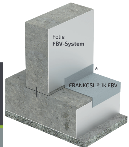
mit Bodenplattenüberstand
